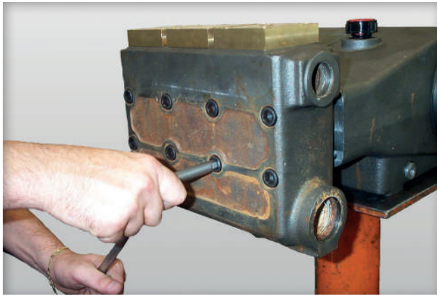
01 Dévisser les 8 vis (pos. 1) du corps de la tête (pos. 2).
