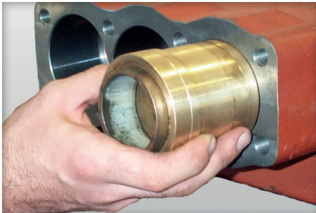
03 Lors du démontage des supports (pos. 3-4) veiller à ne pas endommager les sièges de garniture.
