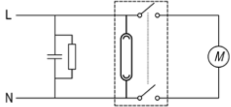
RSV 130 (DRW-13363) 230V 620W
