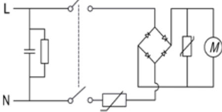
RSAV 200 WD-0361 120V 800W
