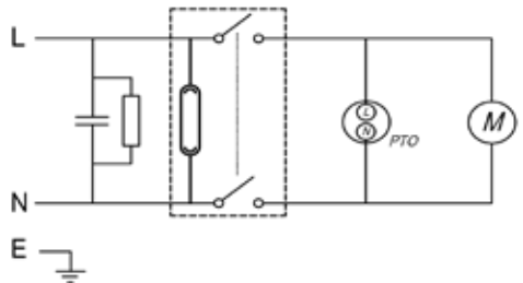
RSV 130 (DRW-13365) 120V 900W
