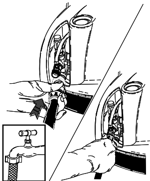
Wasseranschluß
