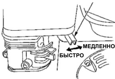
Рычаг-регулятор оборотов
